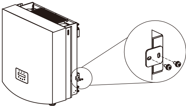
▲ Hình 5.6 Cố định bộ biến tần
