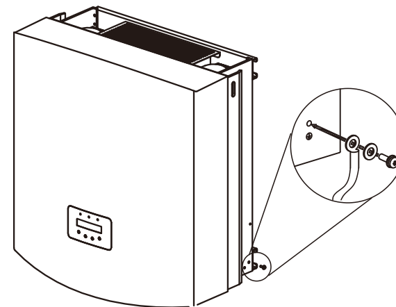
▲ Hình 5.9 Cố định cáp
