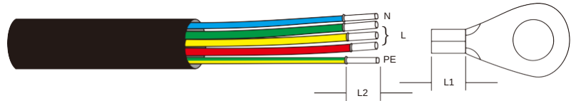
▲ Hình 5.17 Tước vỏ cáp AC
