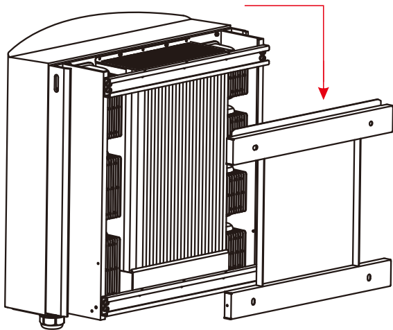
▲ Hình 5.5 Lắp bộ biến tần vào khung lắp
