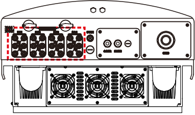
▲ Hình 5.16 Đầu các đầu nối DC với bộ biến tần
