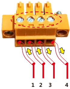
▲ Hình 5.28 Bóc lớp cách điện và kết nối với RS485.
