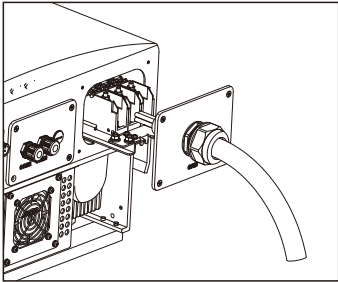
▲ Hình 5.20a Đầu nối cáp với cực nối AC
