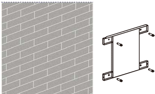
▲ Hình 5.4 Cố định khung lắp vào tường
