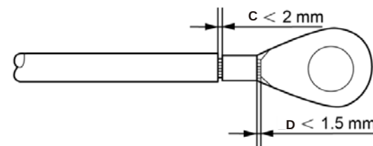
▲ Hình 5.8 Tước vỏ dây
