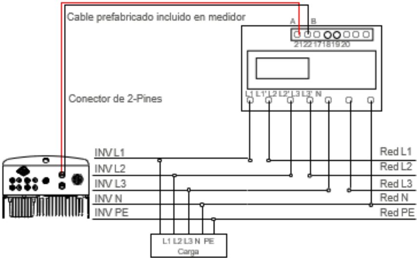
Figura 5.26 Medidor de tipo de inserción directa - "Medidor en la red"
