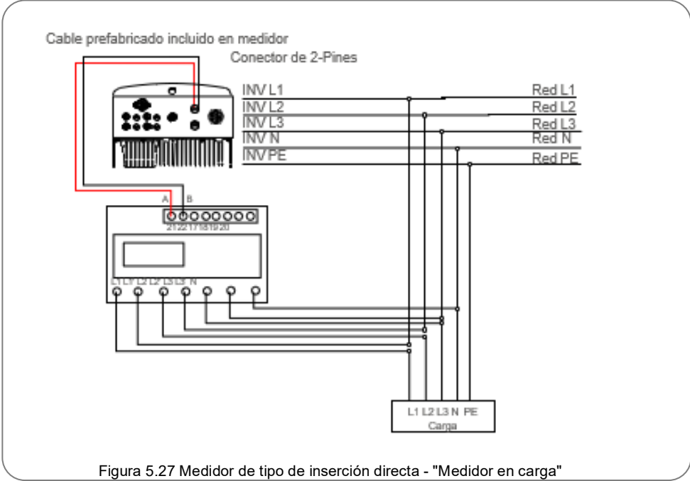
Figura 5.27 Medidor de tipo de inserción directa - "Medidor en carga"
