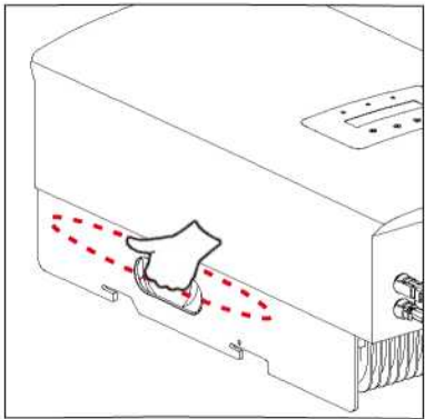
Figura 4.2 Asas del inversor
