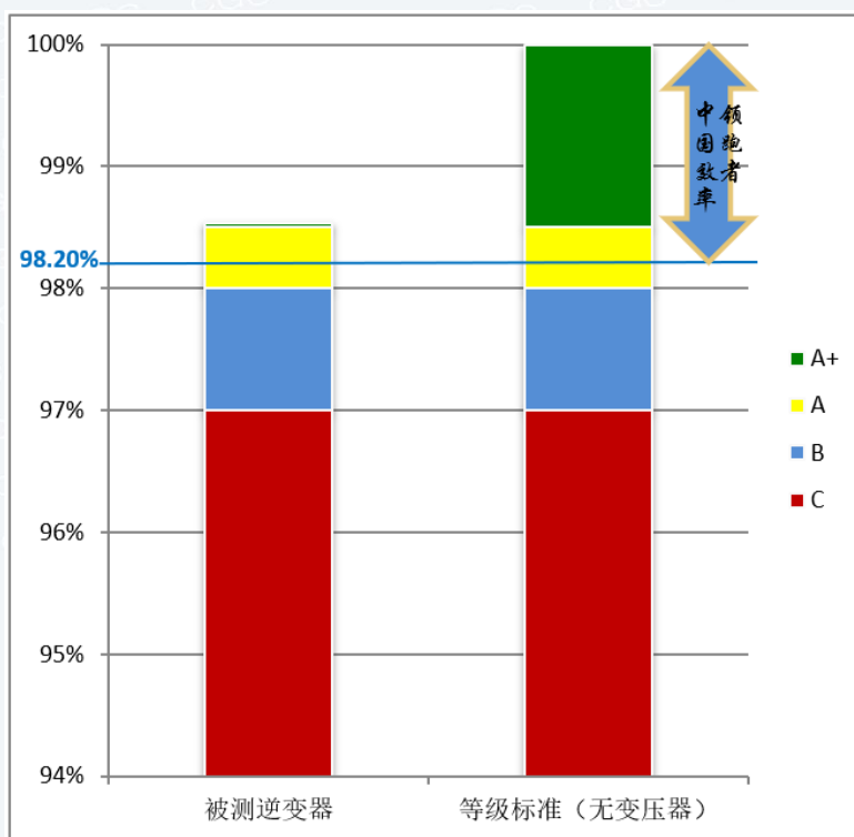
图 1. 逆变器效率水平对比图示
