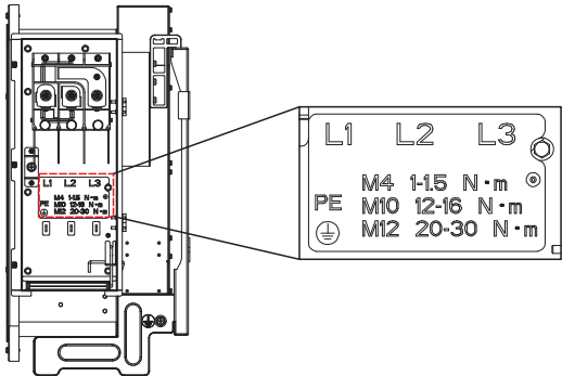
图3.20 交流端子排
