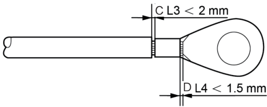
图3.10 线缆压接
