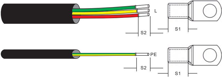
图3.17 剥开交流线缆
