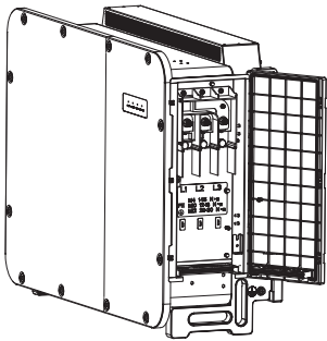
图3.19 拆下接线盒盖
