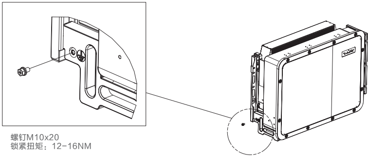
图3.11 固定线缆
