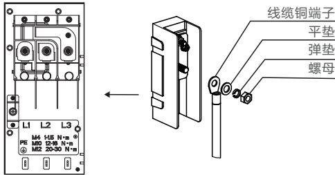
图3.18 铜铝过渡转接端子
