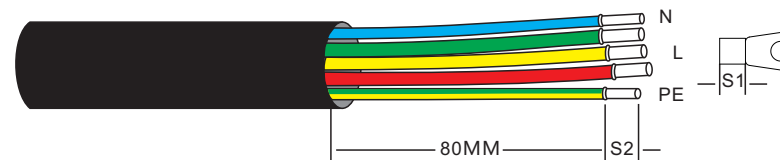
图 5.17 加工电缆线
