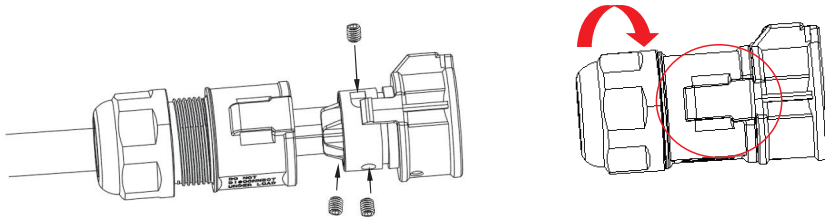
图4.22 连接电缆线
