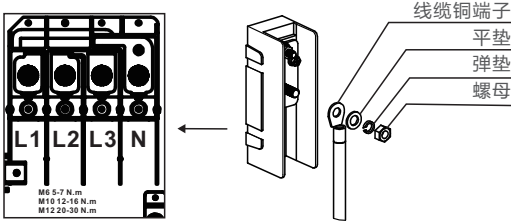
图3.20 铜铝过渡转接端子
