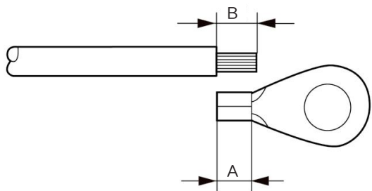
图3.16 剥线长度
