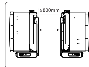
图3.1 逆变器的安装间隙
