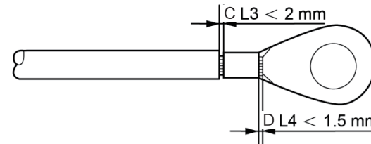
图3.17 线缆压接
