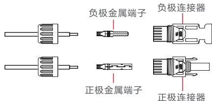
图3.25 拆卸连接器盖螺母
