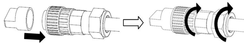
图5.23 组装交流端子
