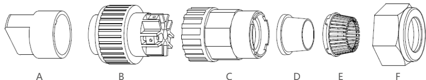
图5.18 交流连接器
