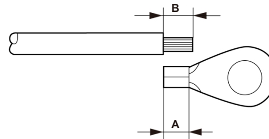
图5.8 剥线长度
