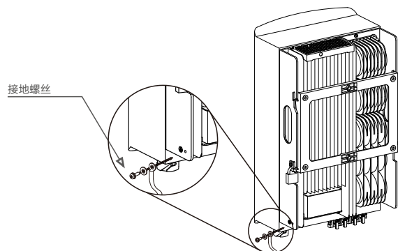
图5.10 线缆固定
