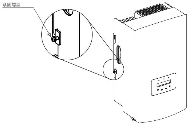
图5.6 固定逆变器
