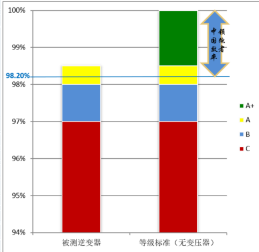
图 1. 逆变器效率水平对比图示
