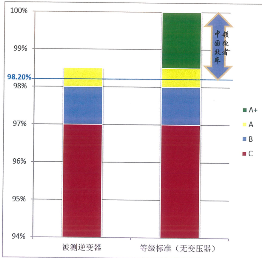
图 1. 逆变器效率水平对比图示
